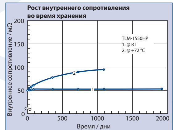
Рис. 3 Рост внутреннего сопротивления во время хранения
