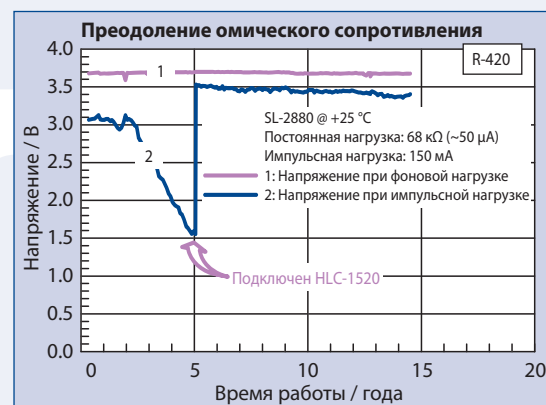
Рис. 1 Преодоление омического сопротивления
