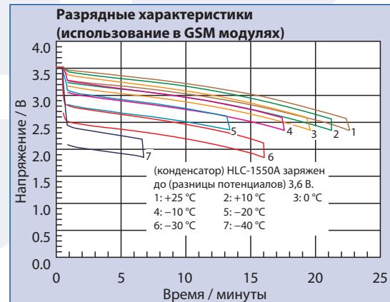
Рис. 2 Разрядные характеристики (использование в GSM модулях)
